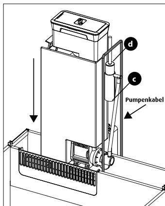
NANO Eiweißabschäumer
